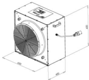
Upper chamber fan 20'
